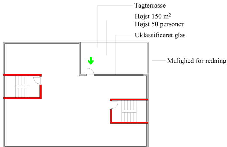
Figur 2.7. Flugtvej fra tagterrasse for undervisningsbygninger i RK3, hvor gulv i øverste etage er højst 9,6 meter over terræn
