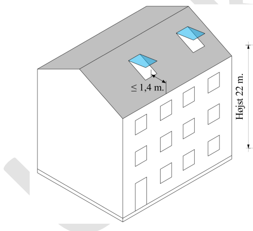
Figur 2.20. Udformning af redningsåbning i tagflade
