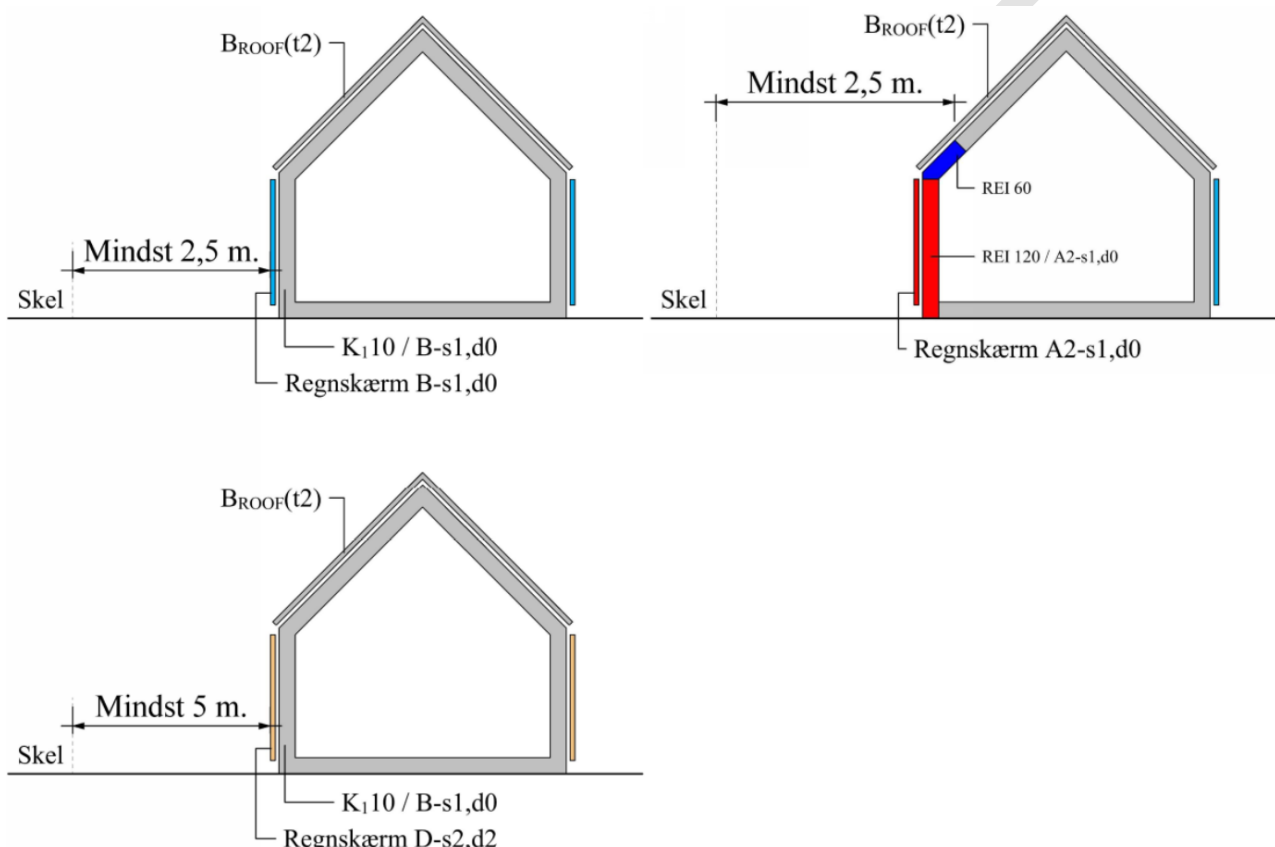
Figur 4.1 Afstande til skel fra undervisningsbygningen ift. udvendig vægoverflade og tagdækning. Alle klassifikationer er minimumskrav.
