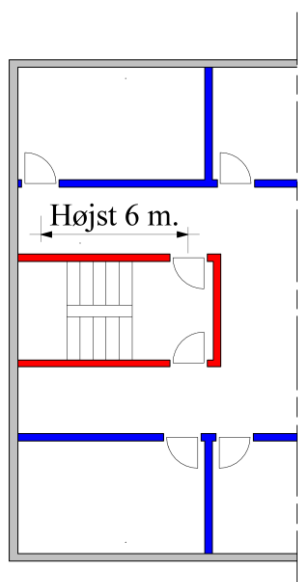
Figur 2.14. Bestemmelse af flugtvej i én retning for en undervisningsetage.
