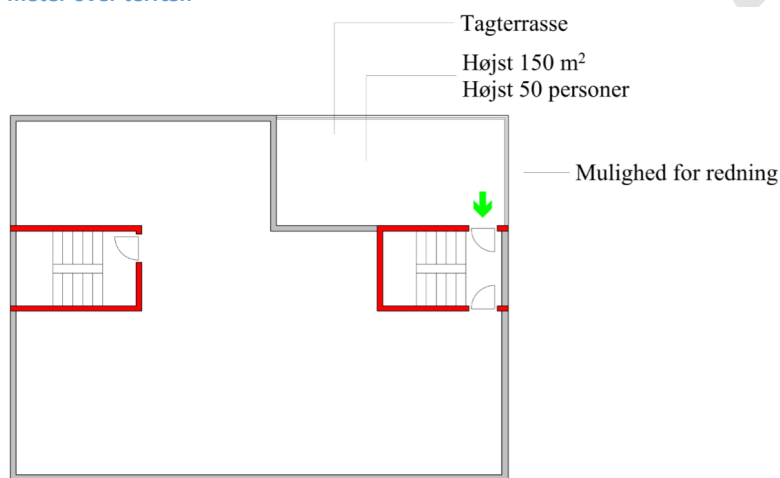
Figur 2.8. Flugtvej fra tagterrasse for undervisningsbygninger i RK3, hvor gulv i øverste etage er højst 22 meter over terræn.
