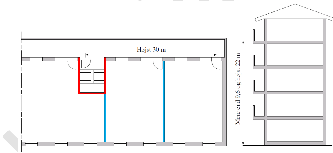
Figur 2.5. Adgang til flugtvejstrappe via altangang for undervisningsbygning, hvor gulv i øverste etage er mellem 9,6 og 22 meter over terræn og redningsberedskabet kan nå enden af altangangen med deres kørbare stiger.
