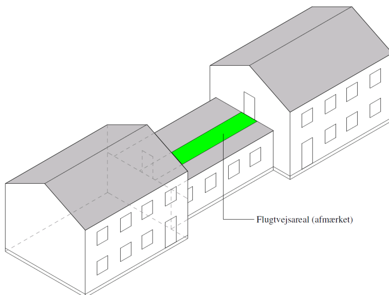
Figur 2.9. Flugtvej over tag for undervisningsbygninger i RK3 med gulv i øverste etage højest 9,6 meter over terræn beregnet til højst 50 personer.
