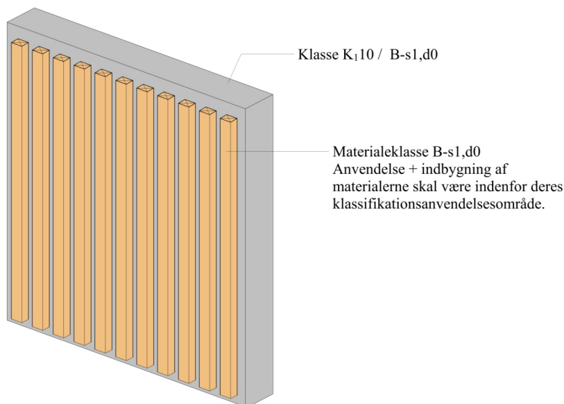
Figur 4.24. Præ-accepterede løsninger på indvendig komplettering i form af listeværk på indvendig beklædning mindst klasse K 1 10 / B-s1,d0 [klasse 1 beklædning]. Alle klassifikationer er minimumskrav.
