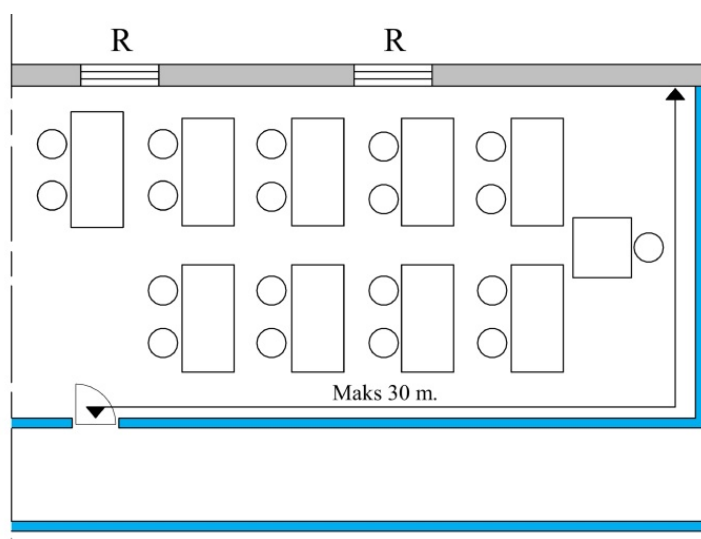
Figur 2.11. Ganglængde i brandcelle med fast og kendt indretning.
