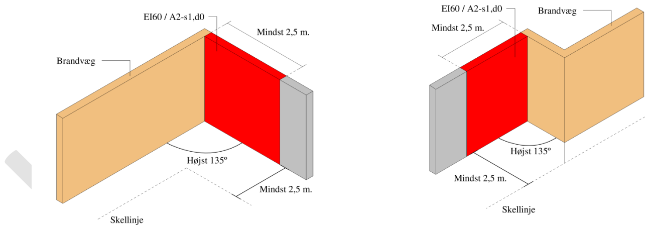
Figur 4.15. Sikring af vandret brandspredning/vinkelsmitte ved brandvæg. Alle klassifikationer er minimumskrav.
