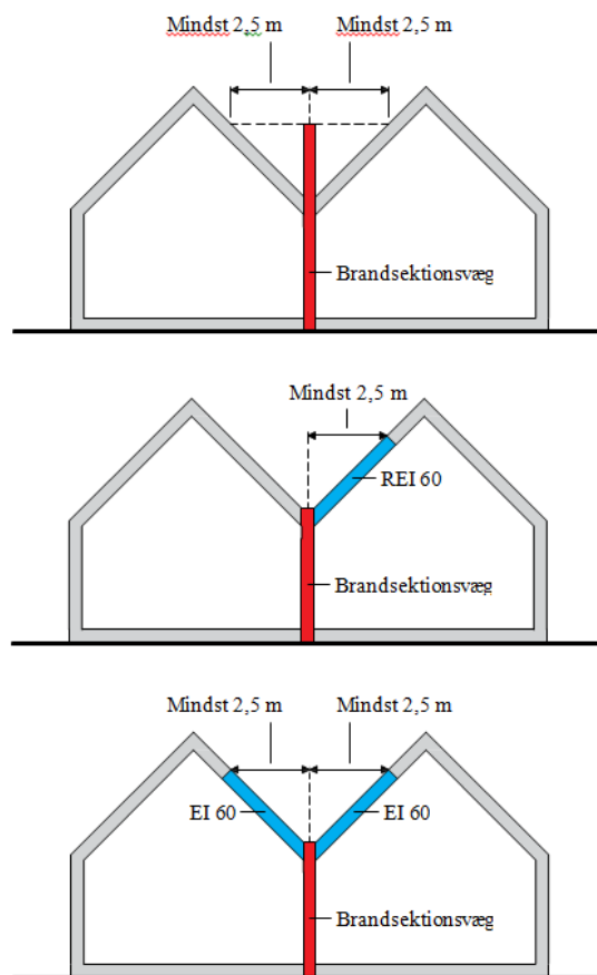
Figur 4.18 Præ-accepterede løsninger for brandkam og brandkamserstatning for undervisningsbygninger med taghældning større end 1:8 mod brandsektionsvæg. Alle klassifikationer er minimumskrav.
