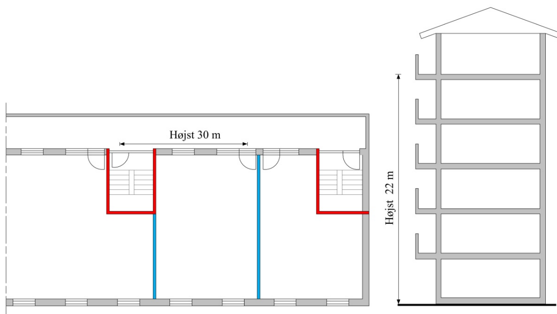
Figur 2.6. Adgang til flugtvejstrappe for undervisningsbygning, hvor redningsberedskabet ikke kan nå altangangen med deres stiger.
