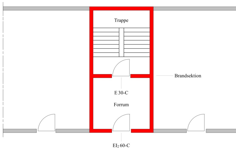
Figur 4.20. Præ-accepteret løsning på en trappe som er ført til kælder i en undervisningsbygning, hvor gulv i øverste etage er højst 22 meter over terræn. Alle klassifikationer er minimumskrav.
