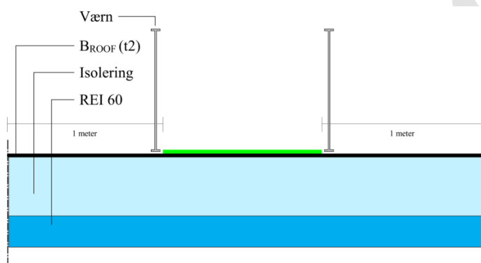
Figur 2.10. Brandmæssig adskillelse under flugtvej over tag. Der må ikke etableres åbninger eller gennemføringer i en afstand af min. 1 meter fra kanten af flugtvejen. Alle klassifikationer er minimumskrav.
