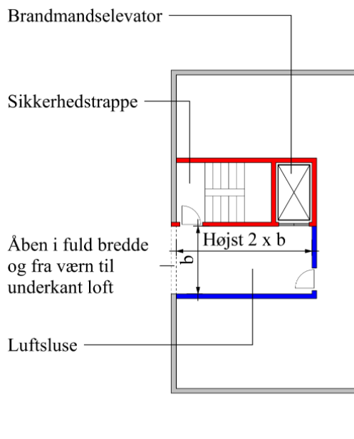
Figur 2.18. Princip for udførelse af luftsluse.
