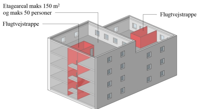
Figur 2.3. Bygningsafsnit hvorfra der kun er adgang til én flugtvejstrappe.
