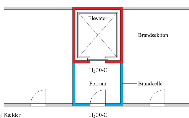
Figur 4.21. Adgang til kælder via forrum fra elevator.
