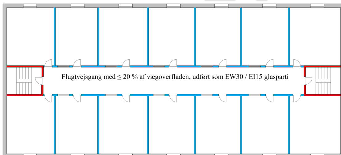
Figur 4.22. Præ-accepterede løsninger på vægadskillelse i flugtvejsgang, hvor op til 20 % af vægoverfladen mellem flugtvejsgang og tilstødende opholdsrum er udført mindst som glasparti klasse EW 30 / EI 15. Alle klassifikationer er minimumskrav.
