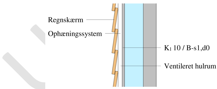
Figur 4.8 Regnskærm uden på ydervæg, med ventileret hulrum. Alle klassifikationer er minimumskrav.
