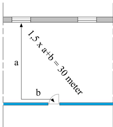
Figur 2.13. Beregning af gangafstand indenfor den brandmæssige enhed til nærmeste flugtvej når indretningen i rummet ikke er kendt.
