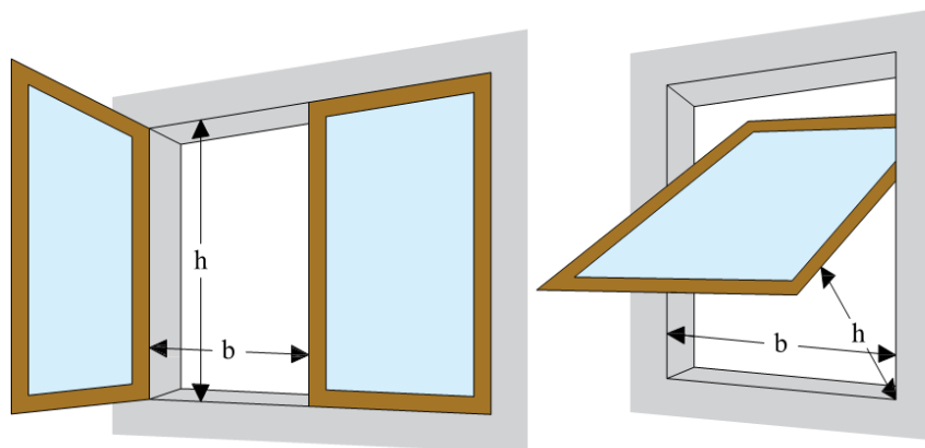
Figur 2.19. Udformning af redningsåbning til personredning.
