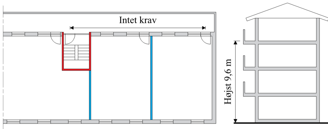
Figur 2.4. Adgang til flugtvejstrappe via altangang for undervisningsbygning, hvor gulv i øverste etage er højst 9,6 meter over terræn og redningsberedskabet kan nå altangangen med deres bærbare stiger.
