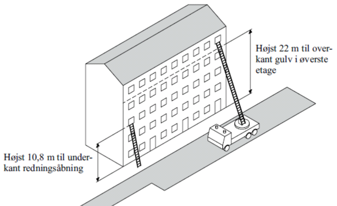
Figur 5.2 præ-accepteret løsning på stigerajsning
