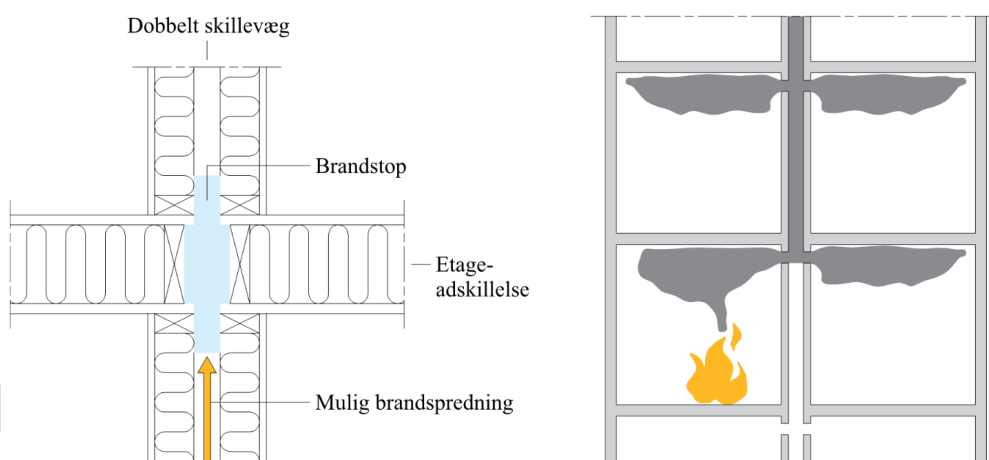
Figur 4.23 Brandstop mellem brandmæssige enheder
